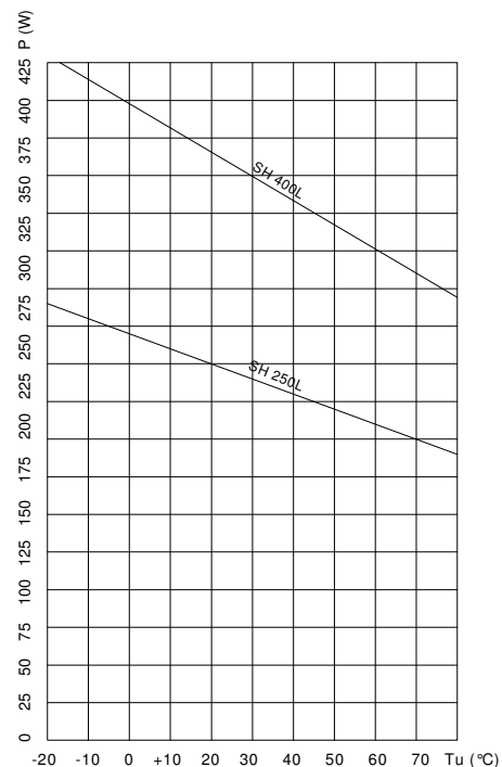
Leistung in Abhängigkeit von der Umgebungstemperatur
