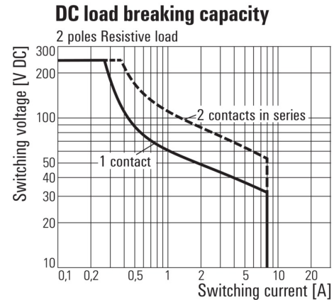
Obciążenie rezystancyjne
