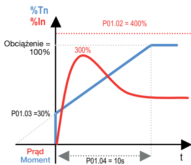
Rozruch w trybie rampy momentu, bez osiągnięcia limitu prądu.
