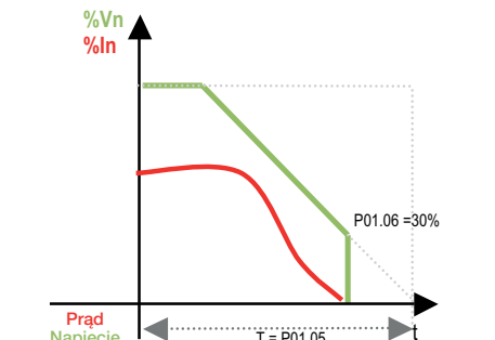
Zatrzymanie w trybie rampy napięcia.
